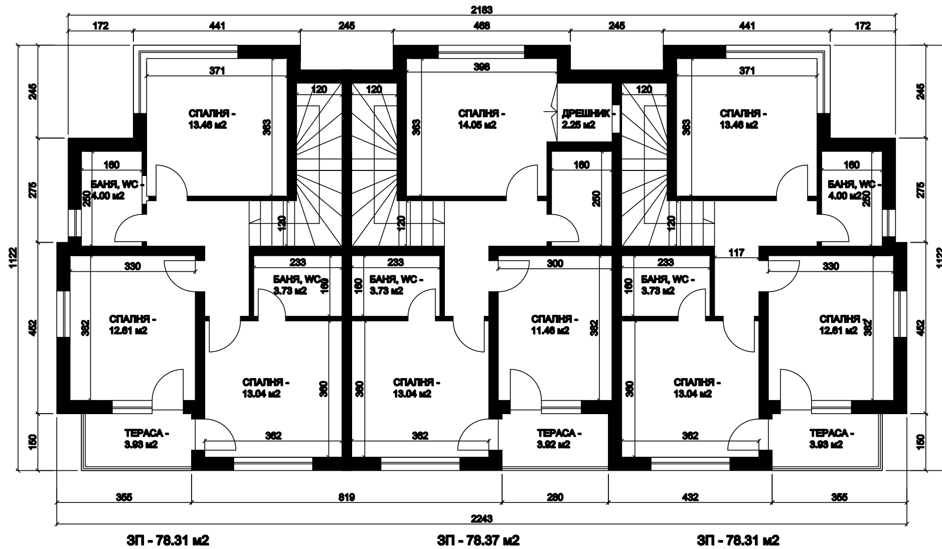
РАЗПРЕДЕЛЕНИЕ ВТОРИ ЕТАЖ М 1:100
